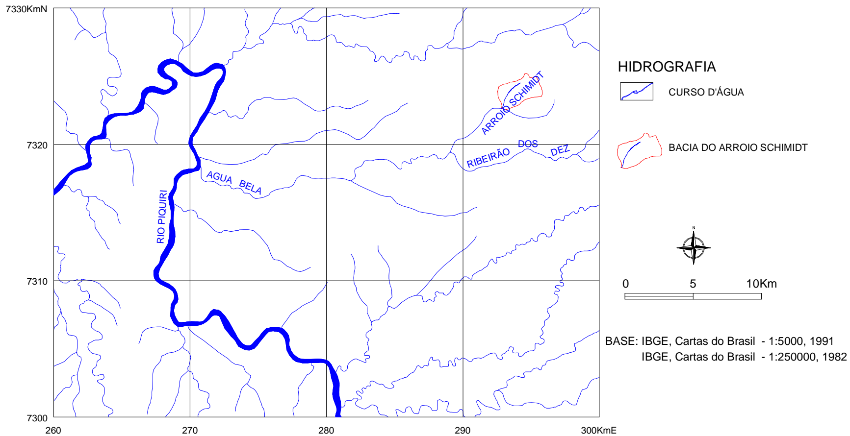
Figura 3: Localização da bacia hidrográfica do Arroio Schmidt, Goioerê - PR
