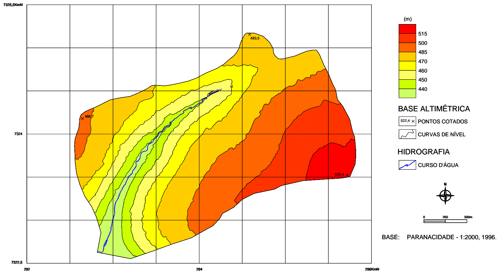
Figura 4: Hipsometria da bacia hidrográfica do Arroio Schimidt, Goioerê - PR
