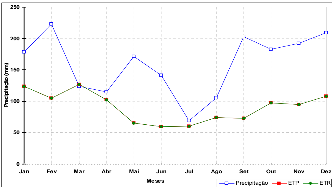
Figura 13: Balanço hídrico normal mensal (1997 – 2002) Fonte: Coagel (2003).
