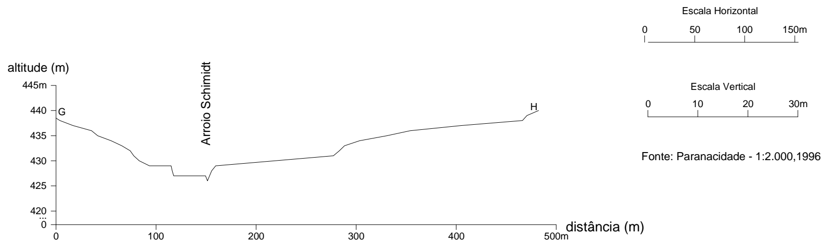
Figura 10: Perfil transversal do baixo curso do Arroio Schmidt
