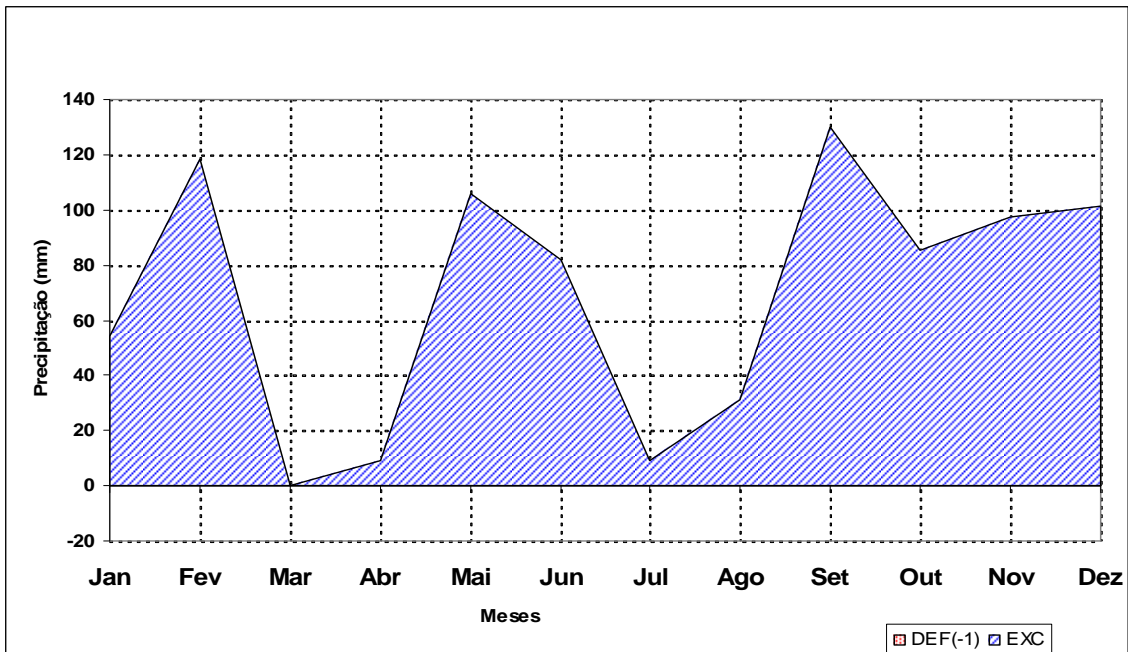
Figura 12: Síntese do balanço hídrico mensal (1997 – 2002) Fonte: Coagel (2003).
