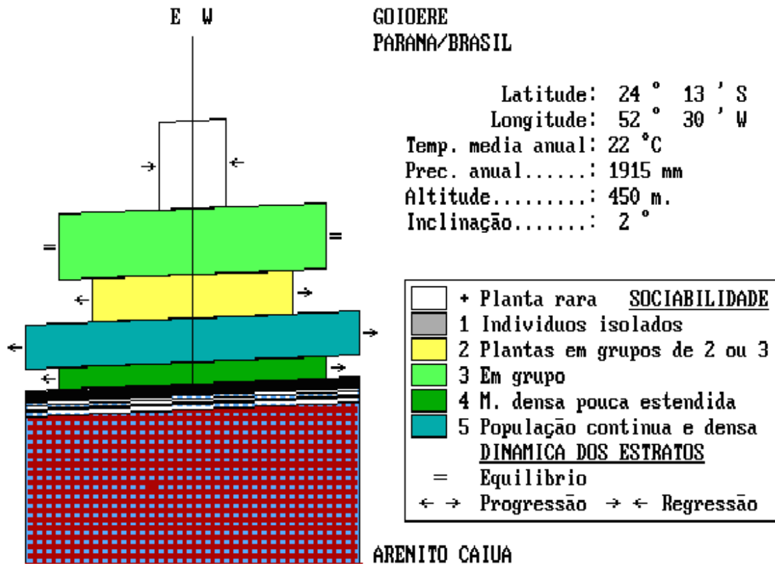
Figura 15: Pirâmide de vegetação da mata nativa próxima a nascente do Arroio Schimidt, Goioerê - PR
