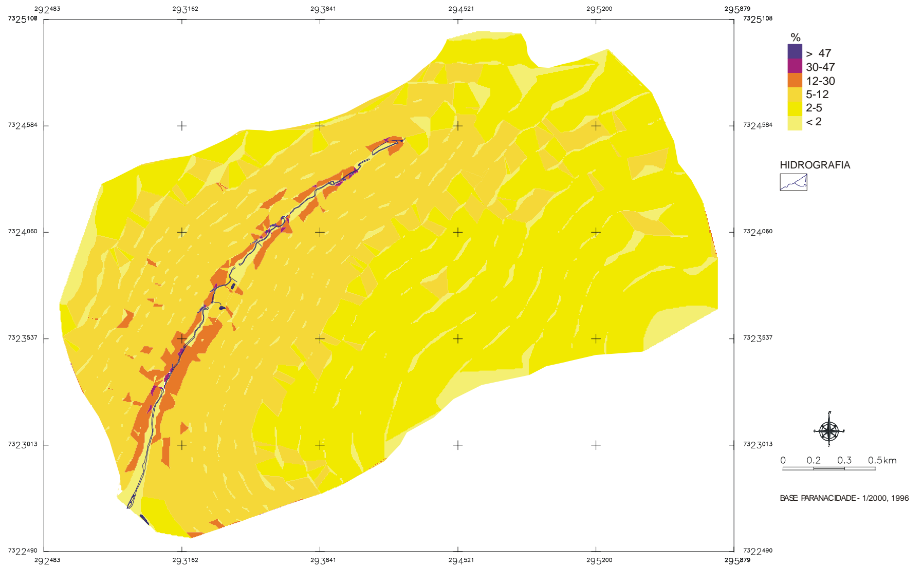
Figura 5: Clinografia da bacia hidrográfica do Arroio Schmidt, Goioerê - PR
