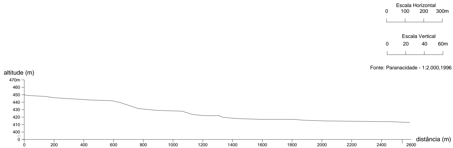
Figura 7: Perfil longitudinal do Arroio Schimidt
