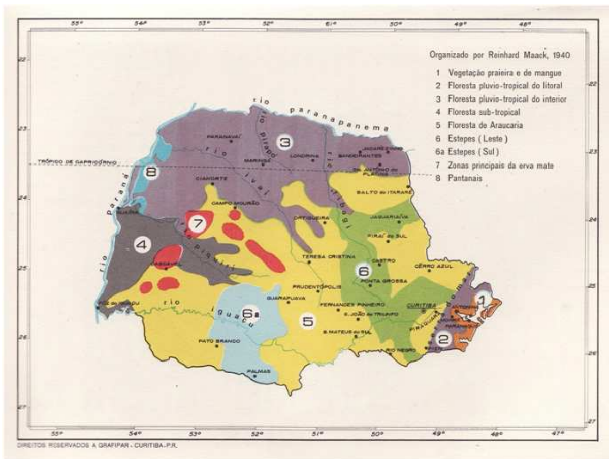
Figura 7- Vegetação do Estado do Paraná organizado por Reinhard Maack no ano de 1940. Fonte: HERTEL, 1969.
