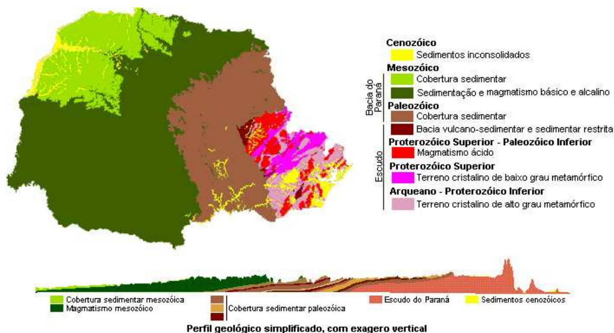
Figura 6- Paraná, principais unidades geológicas do Estado do Paraná Fonte: MINEROPAR, 2003.
