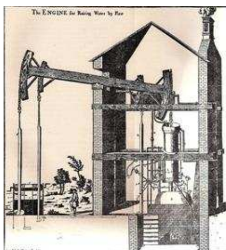
Figura 2- Máquina a vapor de Newcome construída com o fim de mover bombas de água. Fonte: HADDOCK LOBO, 1959.
