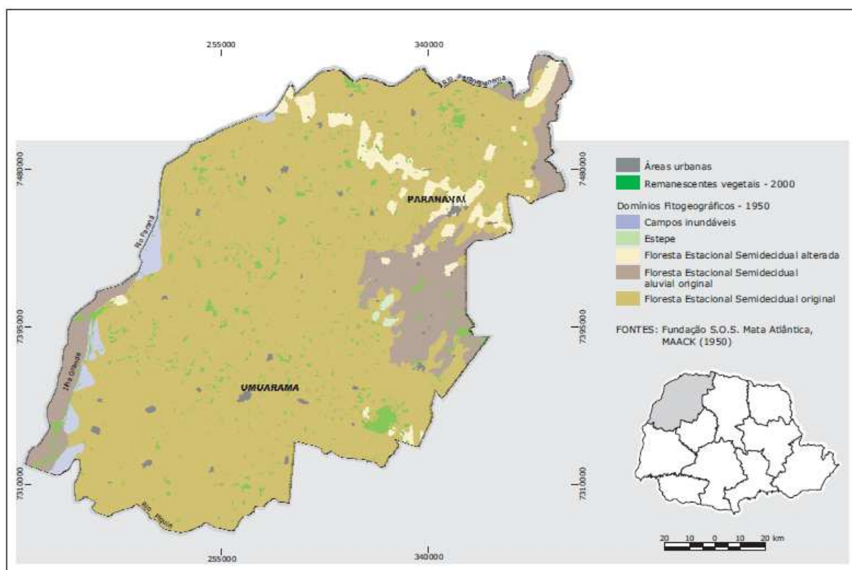
Mapa 7- Estado do Paraná, cobertura vegetal da Mesorregião Noroeste Paranaense. Fonte: IPARDES, 2004.
