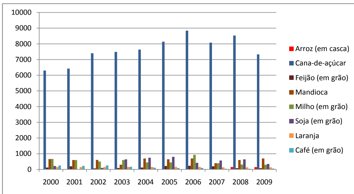
Gráfico 7- Cidade Gaúcha, evolução da área plantada com as principais lavouras- 2000 a 2009.
