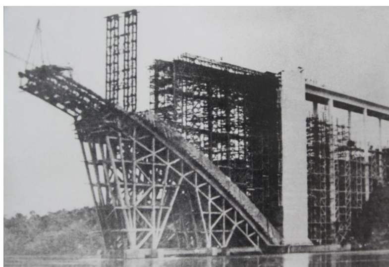
Foto 2: Vista parcial da construção da Ponte Internacional da Amizade, sobre o Rio Paraná: 1956/1965. Fonte: Acervo da Fundação Cultural de Foz do Iguaçu
