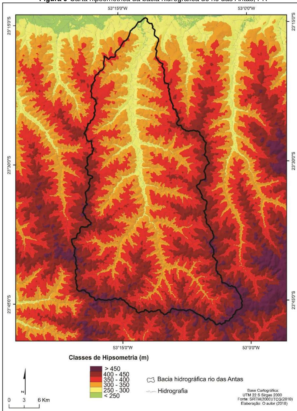
Figura 9 -Carta hipsométrica da bacia hidrográfica do rio das Antas, PR
