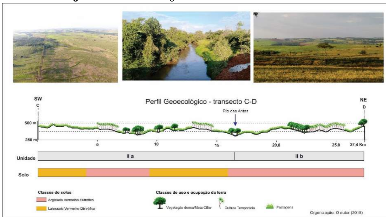
Figura 24- Perfil Geocológico do transecto C-D na unidade II
